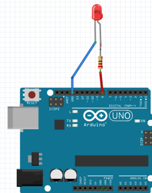
Рис.1. Схема макету. Плата Arduino Uno і світлодіод з резистором 220 Ом.
